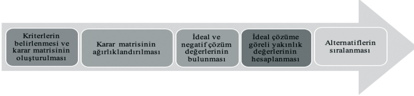
Şekil 6. TOPSIS Yönteminin Adımları (Abdulvahitođlu vd., 2022).
